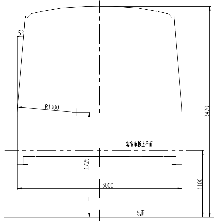
图4 B型车梯形车体轮廓
