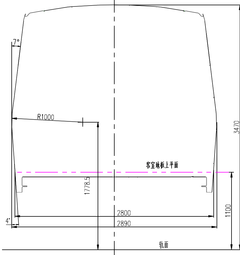
图3 B型车鼓形车体轮廓
