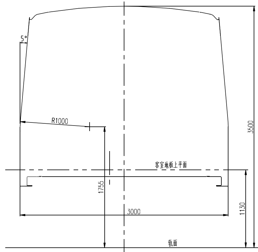
图2 A型车梯形车体轮廓
