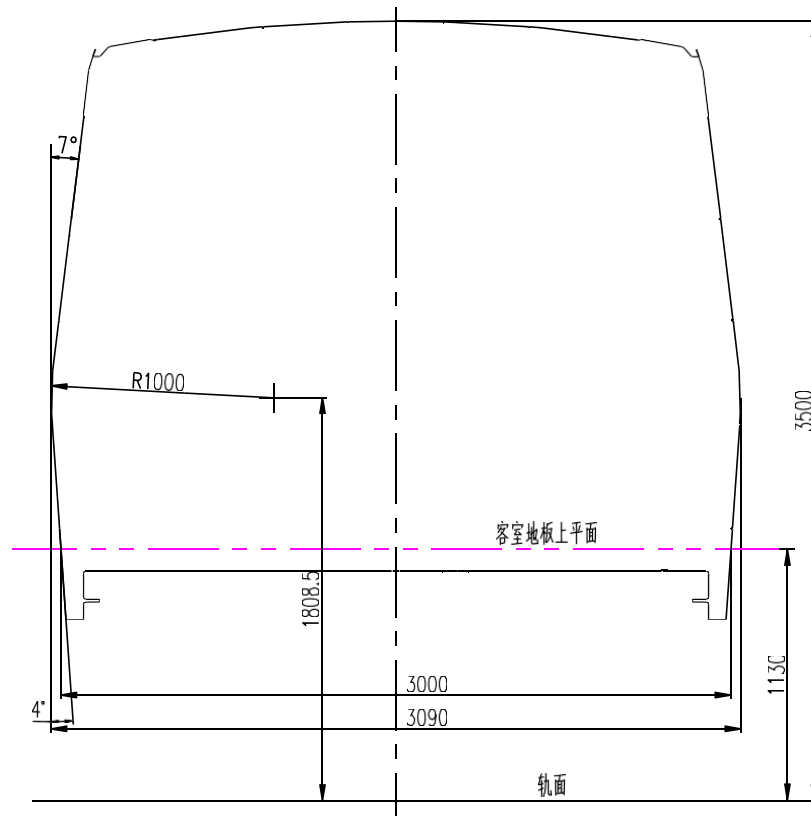
图1 A型车鼓形车体轮廓
